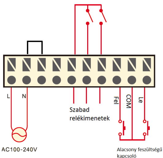
Szabad relé kimenet kiosztása
