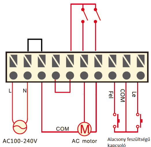
Motor bekötése
